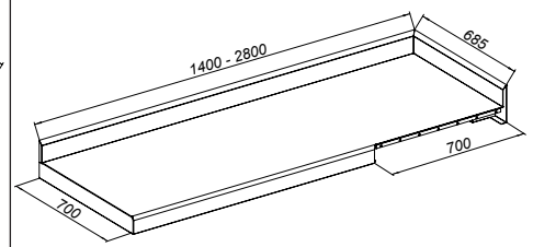
BLPRP-04 - wg rysunku BLPRL-04 - lustrzane odbicie
