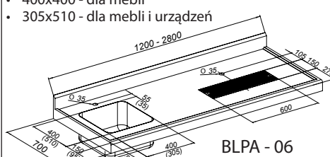
Płyta z zagłębieniem łączona „na włos”
