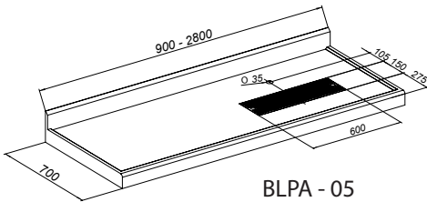
Płyta łączona „na włos”
