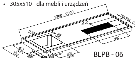
Płyta z zagłębieniem łączona „na włos”
