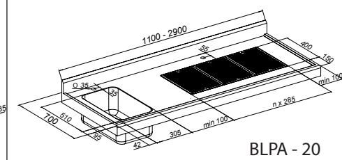
Płyta ze zlewem 307x510 i dużym ociekaczem łączona „na włos” jednostronnie odmiana L (P)
