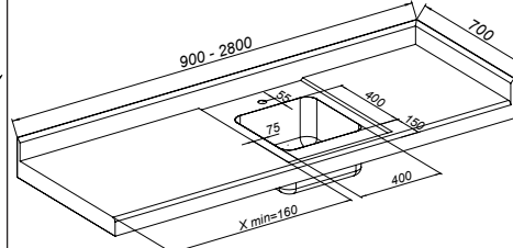
BLPRP-03 - wg rysunku BLPRL-03 - lustrzane odbicie
