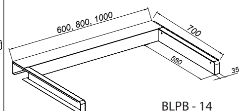
Płyta narożna 90° - zewnętrzna - łączona „na włos” obustronnie
