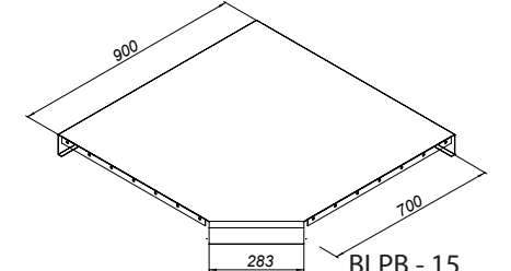
Płyta narożna 45° - zewnętrzna - łączona „na włos” obustronnie
