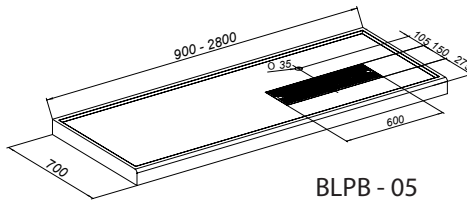
Płyta łączona „na włos”
