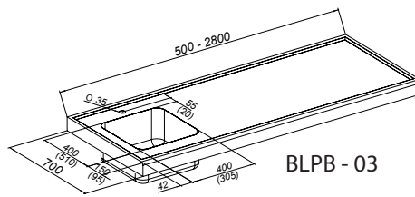
Płyta z ociekaczem, zlewem i otworem pod nalewak do piwa
